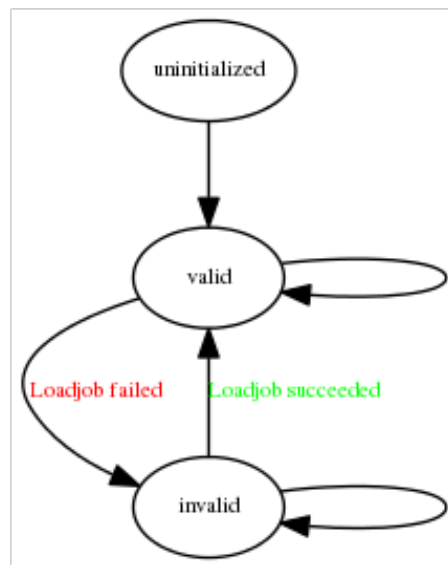
Abbildung 8.3: Zustandsdiagramm einer Resource
