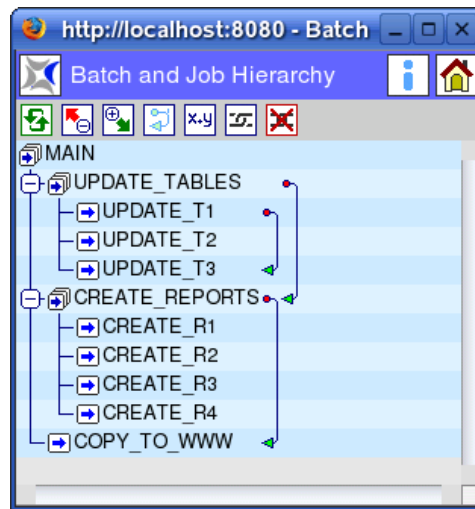
Figure 5: Batchstruktur mit hierarchischer Ordnung nach dem Einbinden des Reports R4
