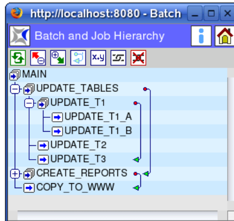
Figure 6: Batchstruktur nach Zerlegung des Prozesses UPDATE_T1 in parallele Teilprozesse
