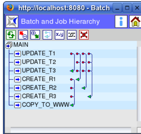
Figure 1: Batchstruktur ohne hierarchische Ordnung
